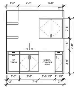
2 WET BAR SCALE: 3/8" = 1'-0"
