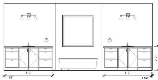
3 PRIMARY BATH SCALE: 3/8" = 1'-0"
